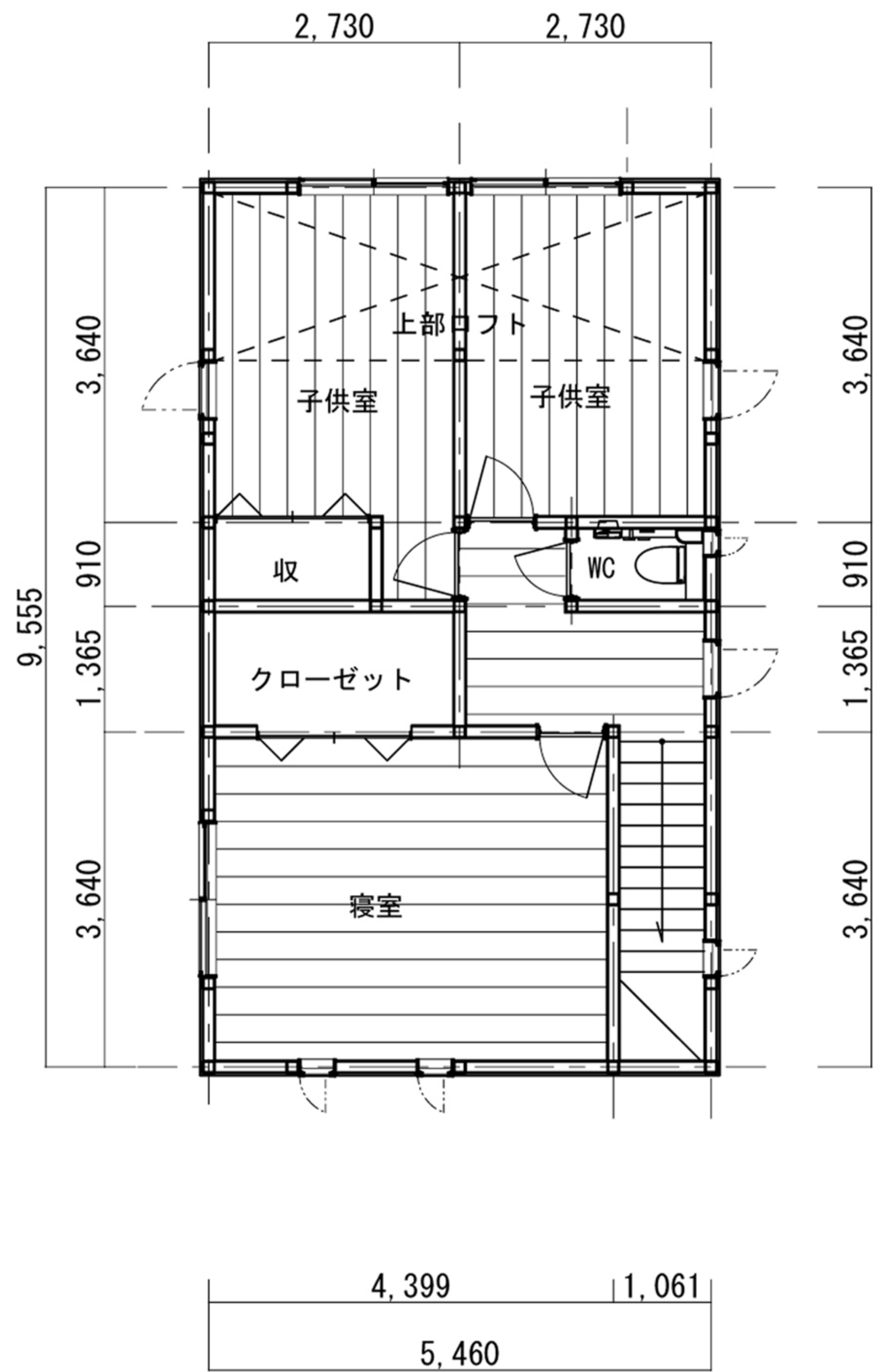
2階平面図 1/100
