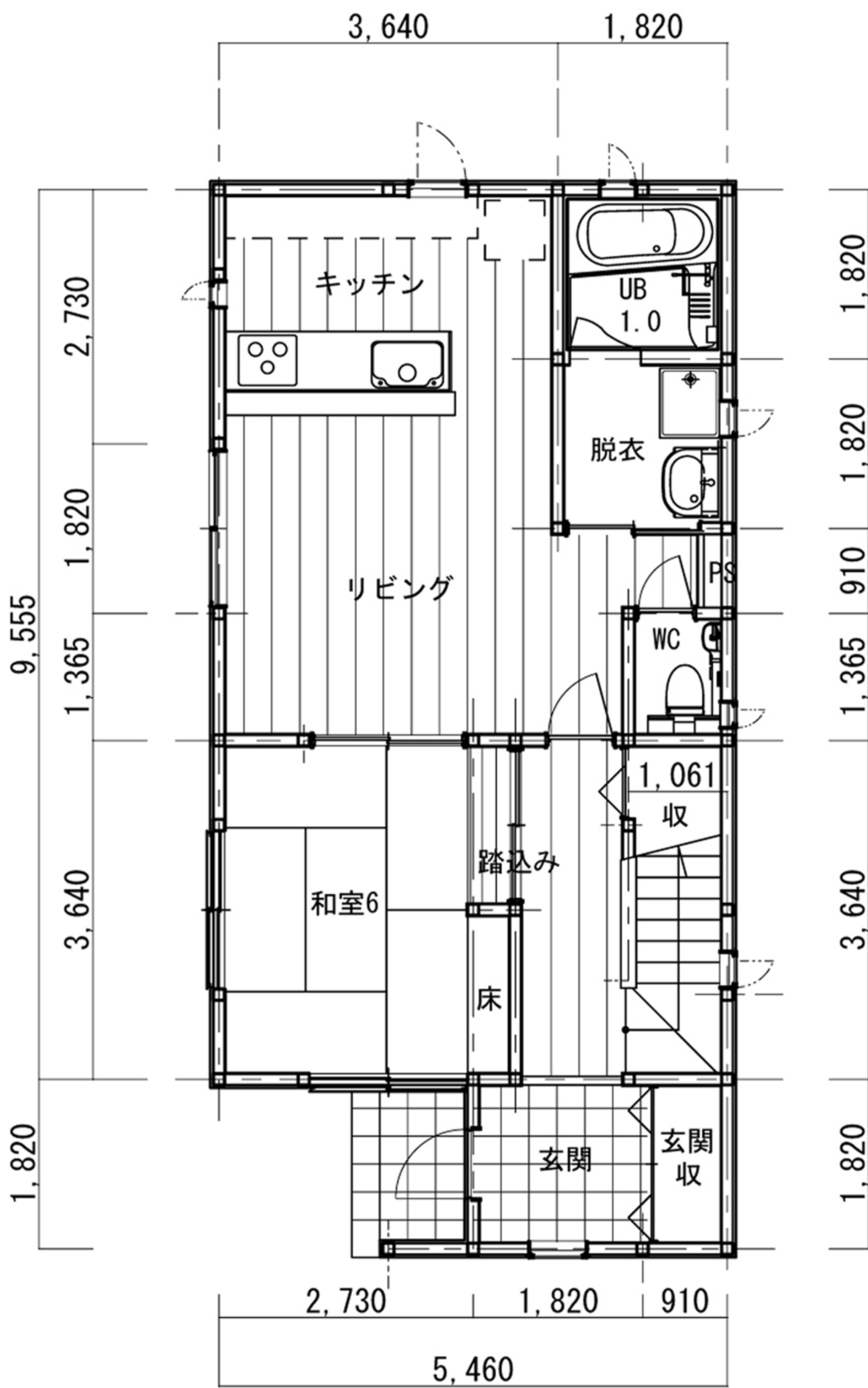
1階平面図 1/100
